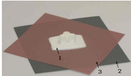
Рисунок 5.4 - Оправка (1), шлифовальная бумага с зернистостью "600" (2), полировальная пленка (3)
