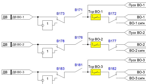
Рисунок 4.2.7 – Функциональная схема внешнего отключения
