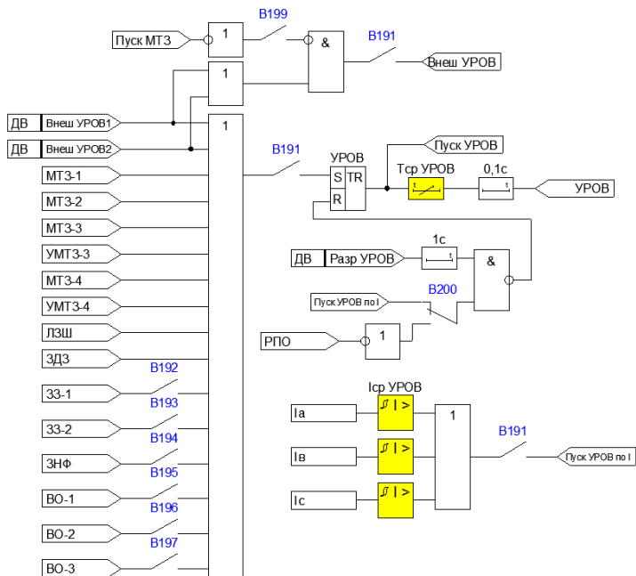
Рисунок 4.2.6 – Функциональная схема УРОВ
