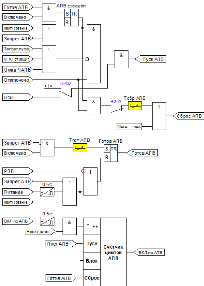
Рисунок 4.2.5 – Функциональная схема АПВ
