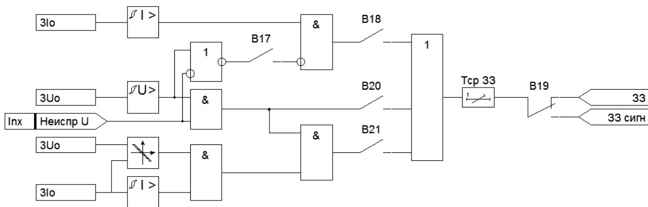
Рисунок 1.6.3 – Функциональная схема ЗЗ
