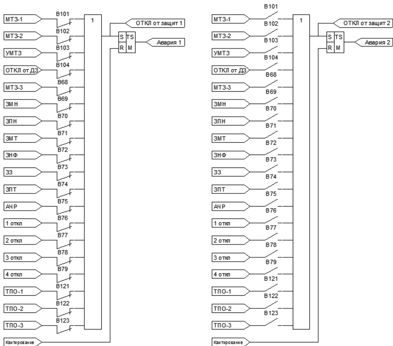
Рисунок 1.6.18.а – Функциональная схема формирования сигналов «Авария 1» и «Авария 2» МКЗП-ОТ
