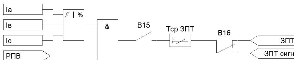
Рисунок 1.6.6 – Функциональная схема ЗПТ
