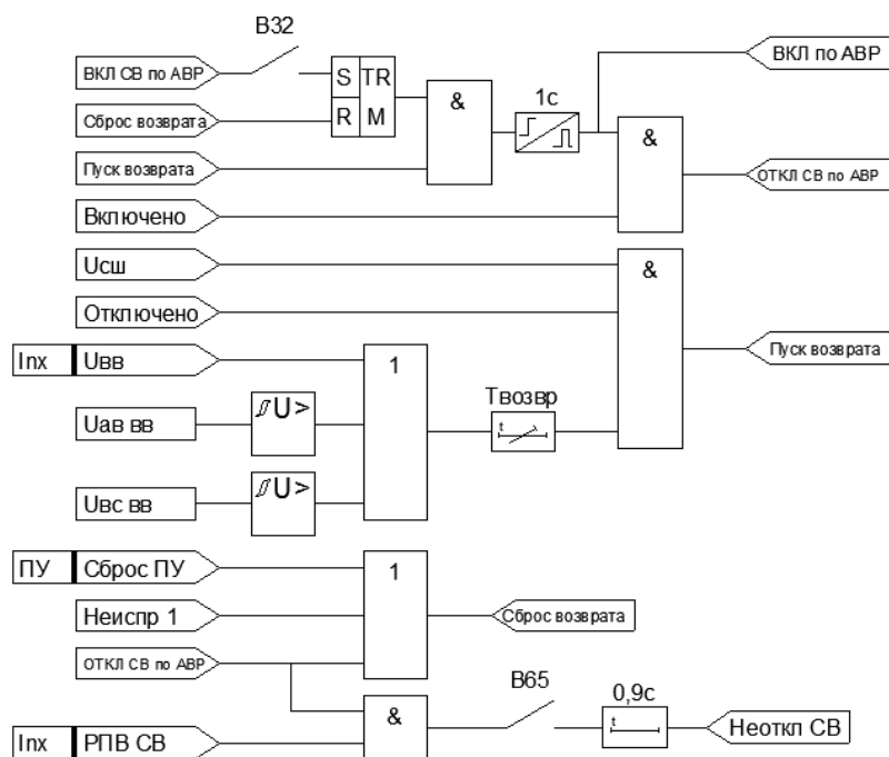
Рисунок 1.6.25 – Функциональная схема возврата после АВР
