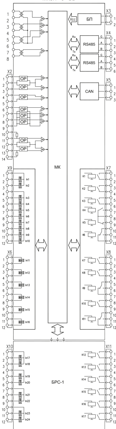
Рисунок Б.2 – Внешние цепи ВВ
