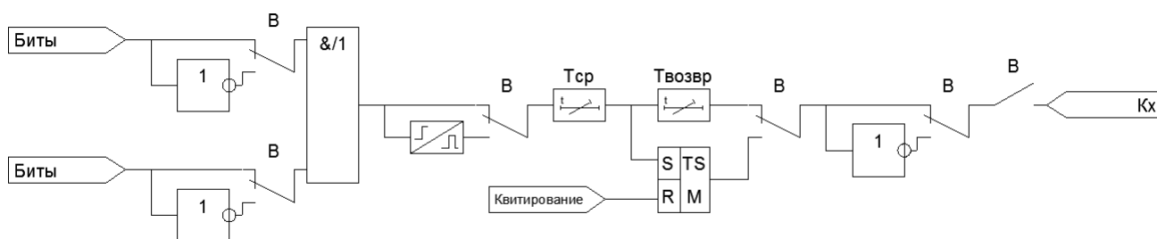
Рисунок 1.6.20 – Функциональная схема логики свободно программируемых реле
