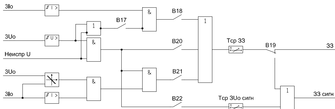
Рисунок 1.6.5 – Функциональная схема ЗЗ
