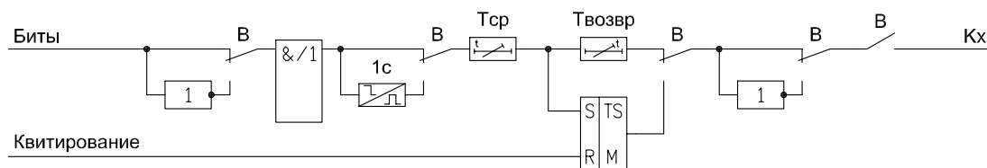
Рисунок 1.6.25 – Функциональная схема логики свободно программируемого реле
