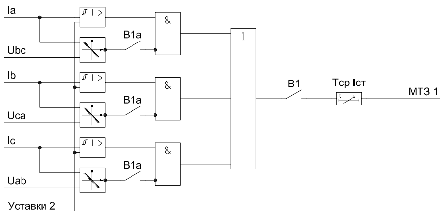
Рисунок 1.6.1 – Функциональная схема МТЗ-1
