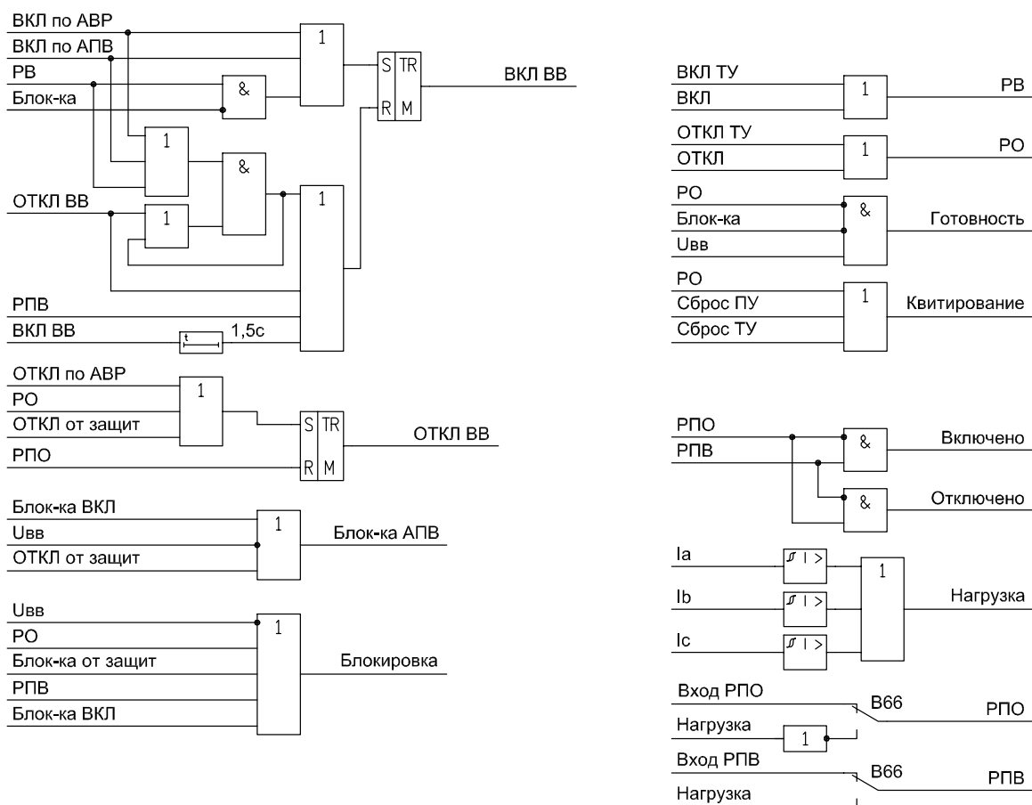
Рисунок 1.6.21 – Функциональная схема логики управления выключателем
