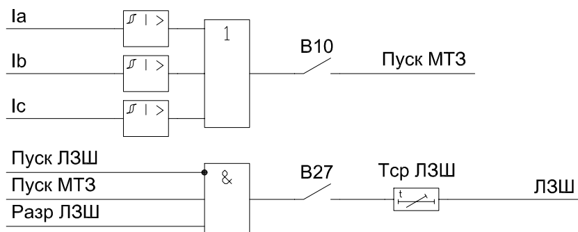
Рисунок 1.6.12 – Функциональная схема пускового органа ЛЗШ
