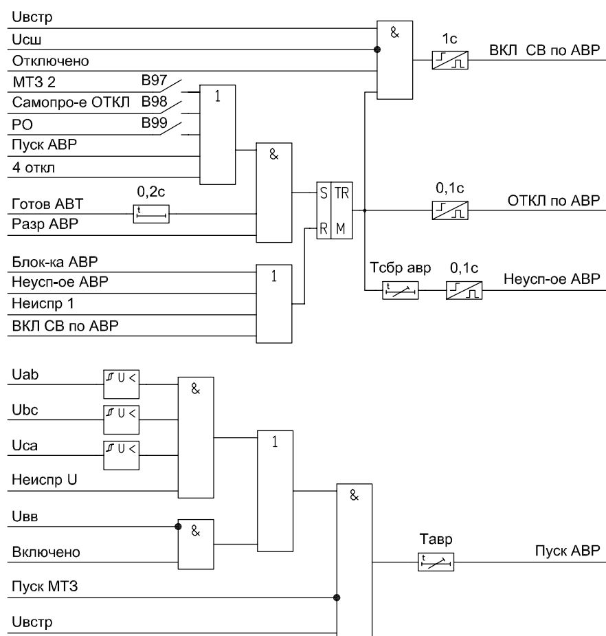
Рисунок 1.6.18 – Функциональная схема АВР
