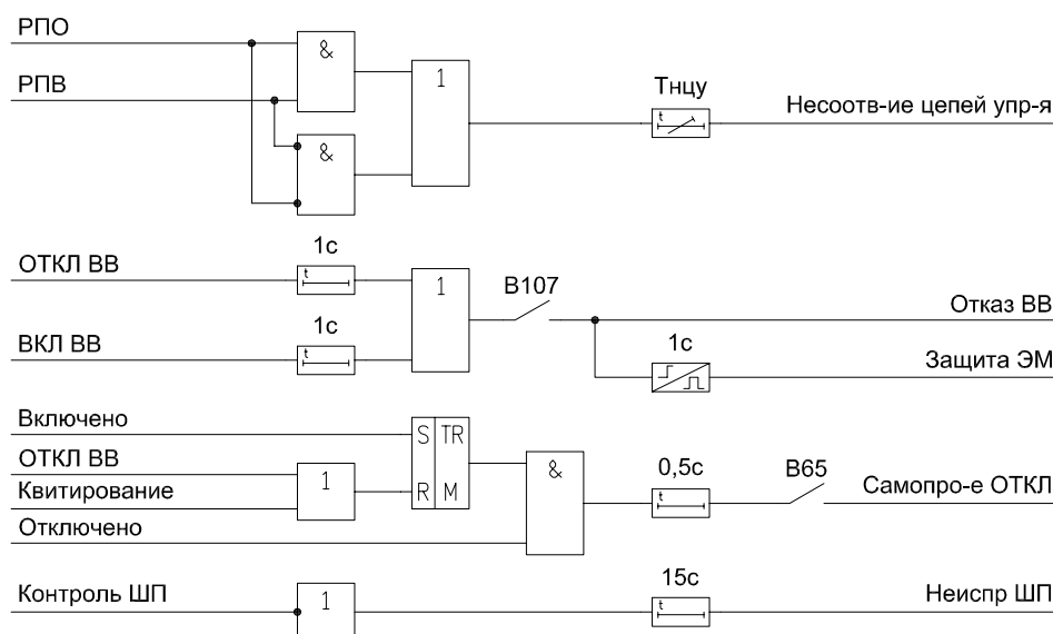
Рисунок 1.6.22 – Функциональная схема логики диагностики выключателя
