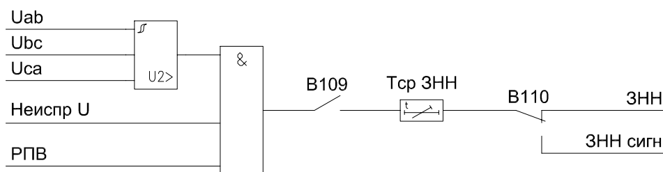
Рисунок 1.6.11 – Функциональная схема ЗНН
