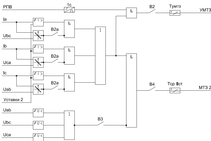
Рисунок 1.6.2 – Функциональная схема МТЗ-2
