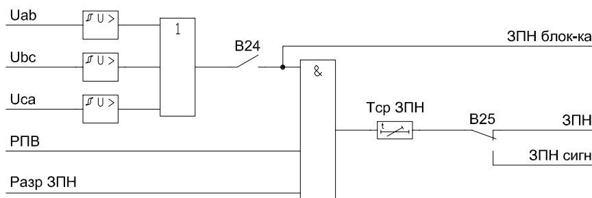
Рисунок 1.6.10 – Функциональная схема ЗПН
