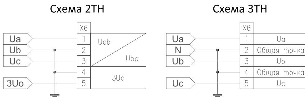
Рисунок 1.5.1 – Варианты подключения цепей напряжения
