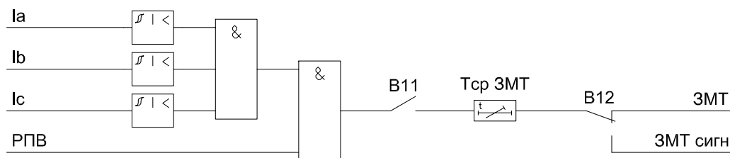
Рисунок 1.6.7 – Функциональная схема ЗМТ
