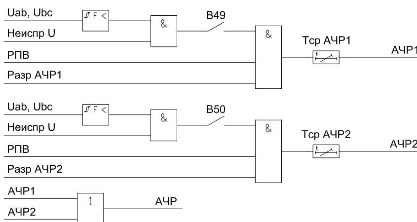
Рисунок 1.6.16 – Функциональная схема АЧР
