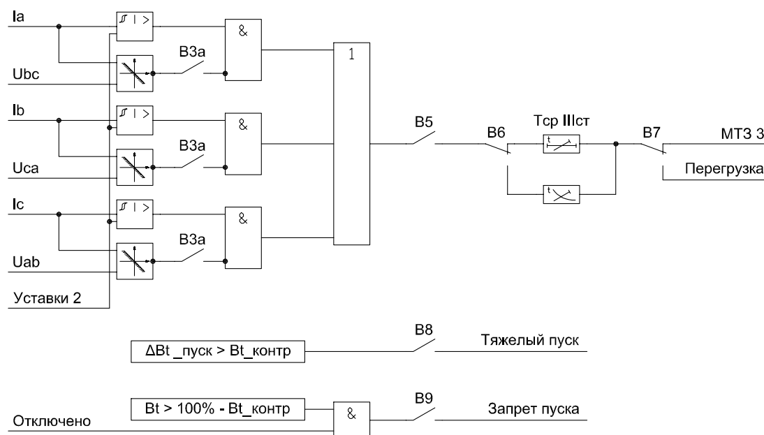
Рисунок 1.6.3 – Функциональная схема МТЗ-3
