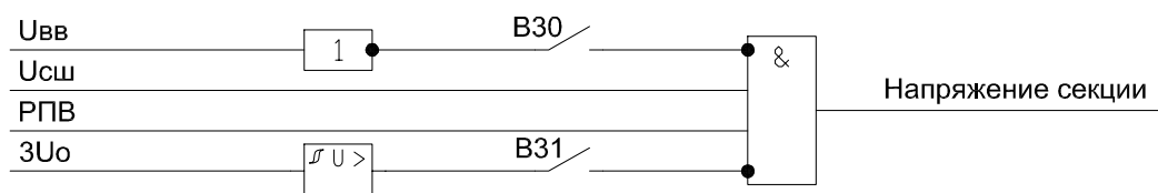
Рисунок 1.6.19 – Функциональная схема формирования сигнала «Увстр» для соседней секции шин
