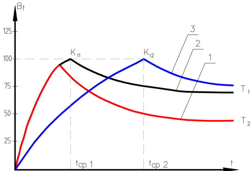
Рисунок 1.6.4 – Зависимости B_t = f(t) при различных кратностях тока K_I : 1 – зависимость B_t = f(t) при кратности тока перегрузки K_{I1} и устранении перегрузки до момента отключения электродвигателя; 2 – зависимость B_t = f(t) при кратности тока перегрузки K_{I1} и отключении электродвигателя при достижении B_t = 100 ; 3 – зависимость B_t = f(t) при кратности тока перегрузки K_{I2} и отключении электродвигателя.
