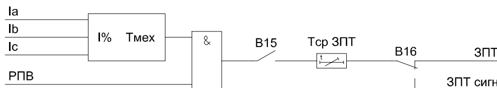
Рисунок 1.6.8 – Функциональная схема ЗПТ
