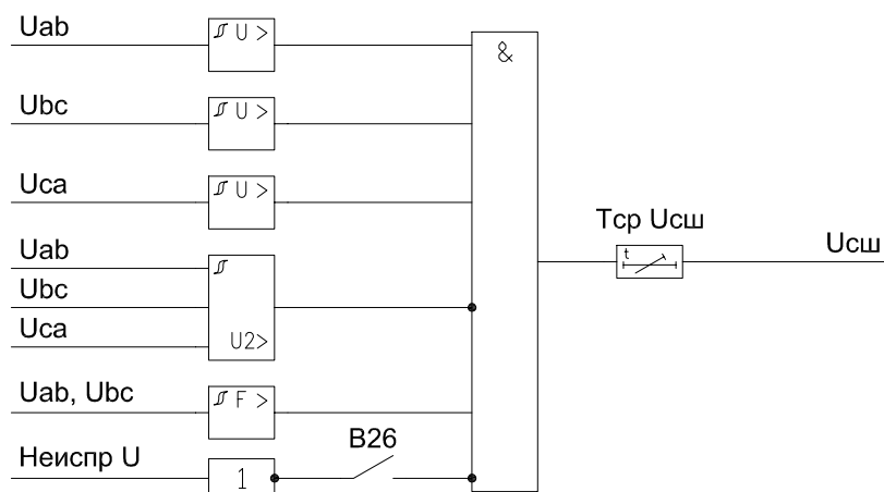
Рисунок 1.6.17 – Функциональная схема формирования U_{сш}
