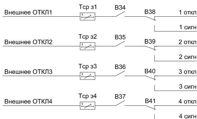
Рисунок 1.6.15 – Функциональная схема отключений от внешних защит
