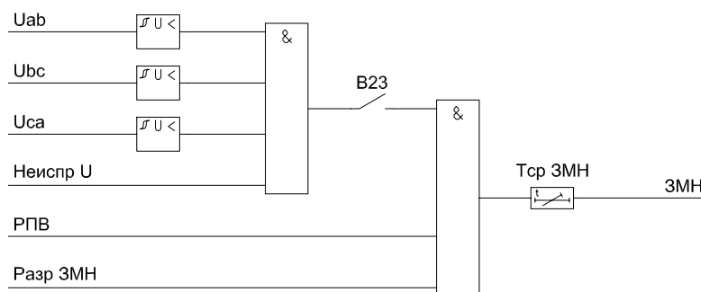
Рисунок 1.6.9 – Функциональная схема ЗМН
