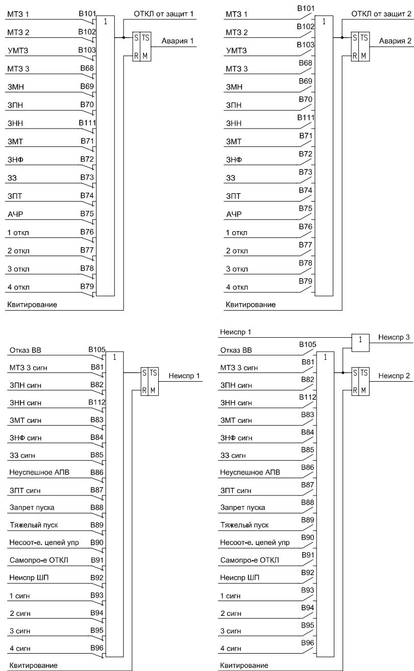
Рисунок 1.6.23 – Функциональная схема формирования сигналов «Авария 1», «Авария 2», «Неиспр 1» и «Неиспр 2»
