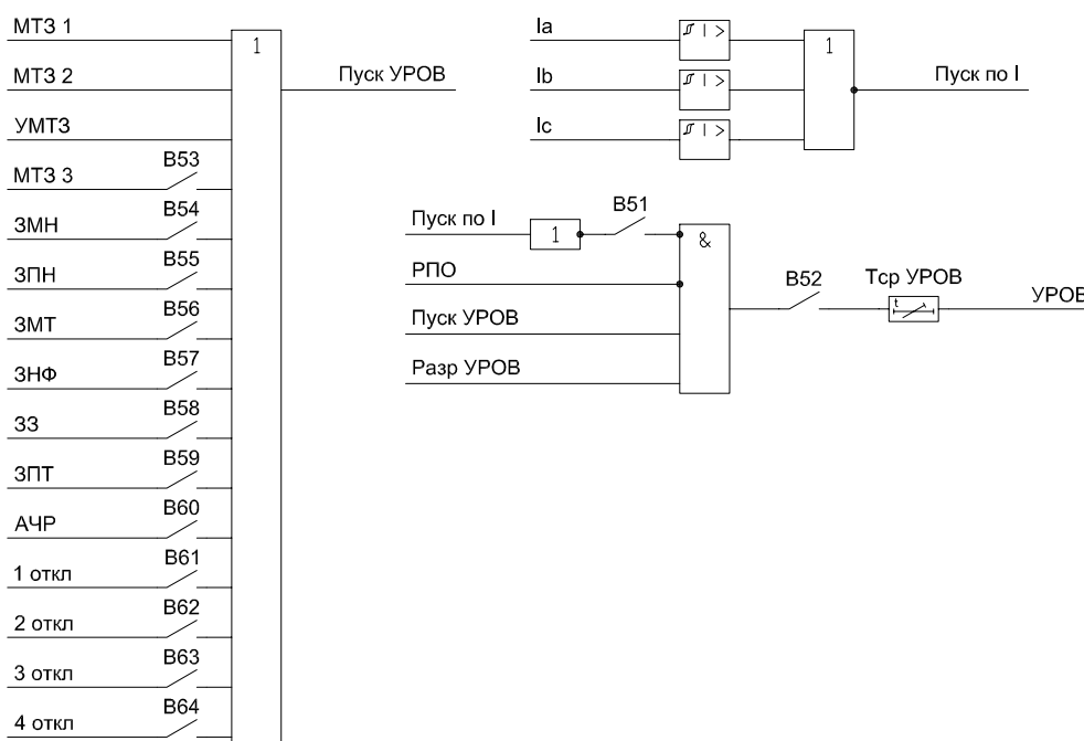
Рисунок 1.6.14 – Функциональная схема УРОВ
