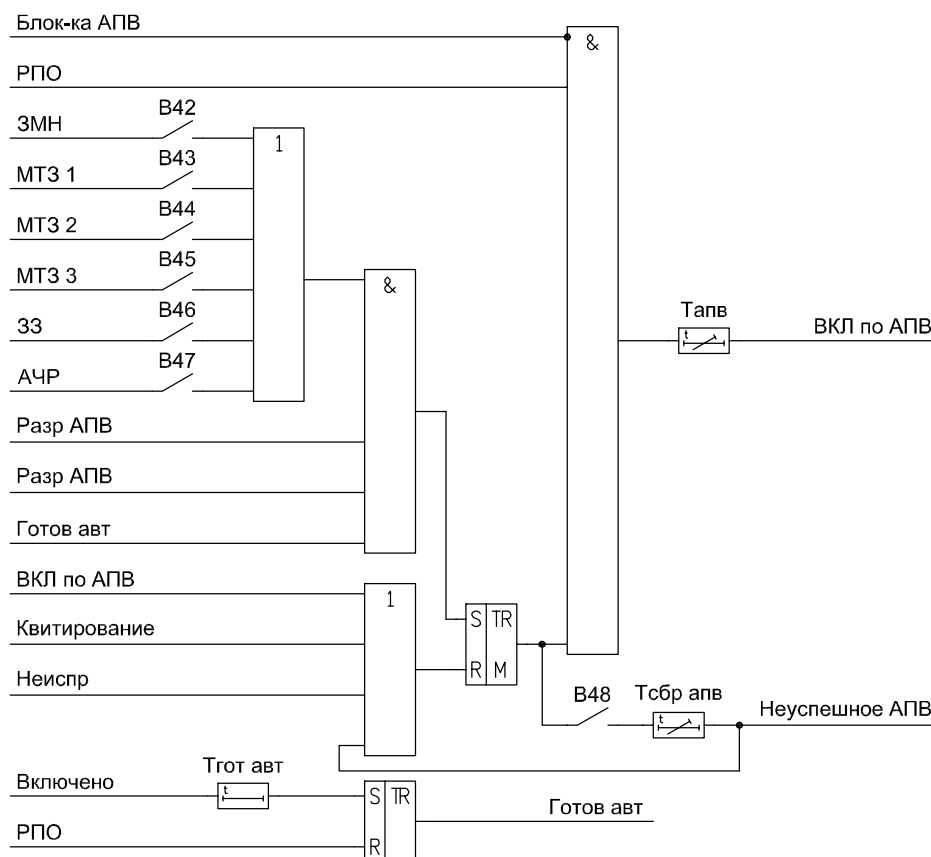
Рисунок 1.6.13 – Функциональная схема АПВ
