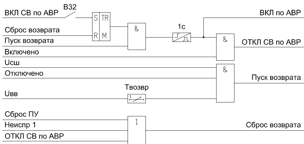
Рисунок 1.6.20 – Функциональная схема возврата после АВР
