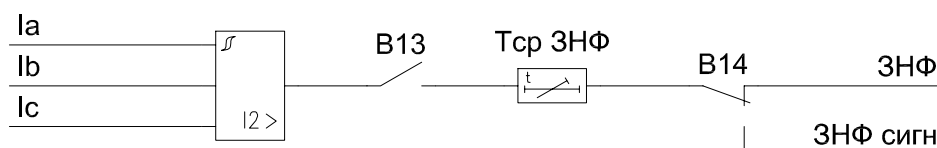
Рисунок 1.6.6 – Функциональная схема ЗНФ
