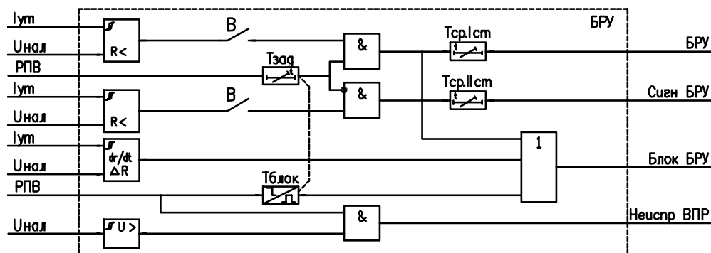
Рисунок 1.6.12 – Функциональная схема БРУ
