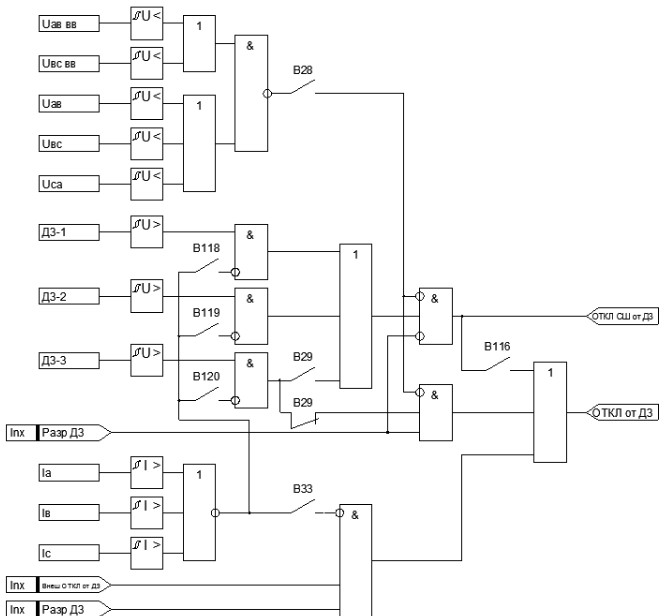
Функциональная схема ДЗ для вводного присоединения
