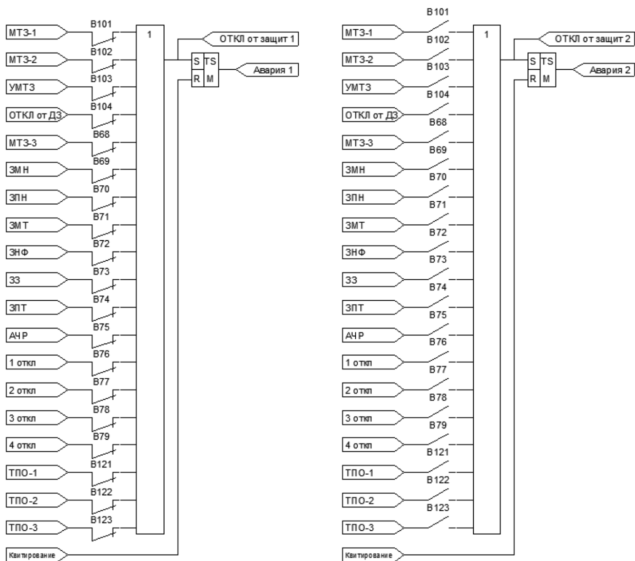
Рисунок 1.6.18.а – Функциональная схема формирования сигналов «Авария 1» и «Авария 2» МКЗП-ОТ
