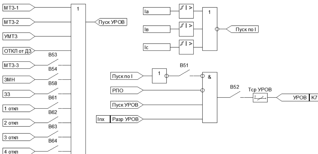
Рисунок 1.6.22 – Функциональная схема УРОВ ВВ
