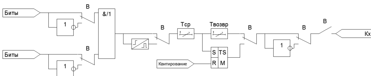
Рисунок 1.6.20 – Функциональная схема логики свободно программируемых реле
