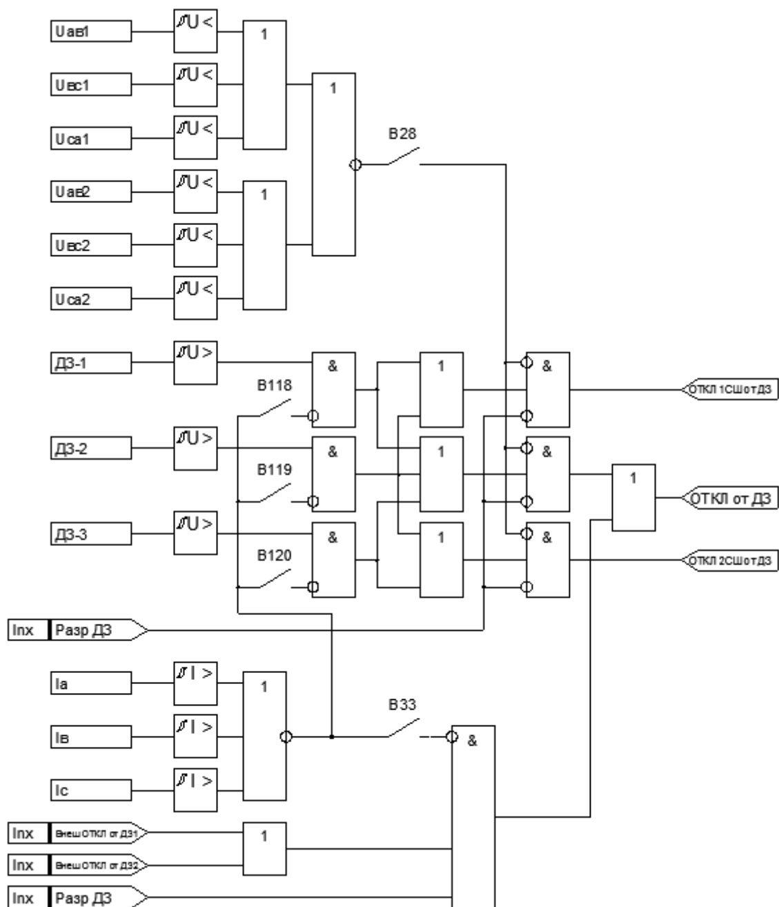
Рисунок 1.6.10 (окончание) – Функциональная схема ДЗ для секционного выключателя
