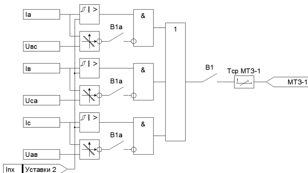
Рисунок 1.6.1.а – Функциональная схема МТЗ-1
