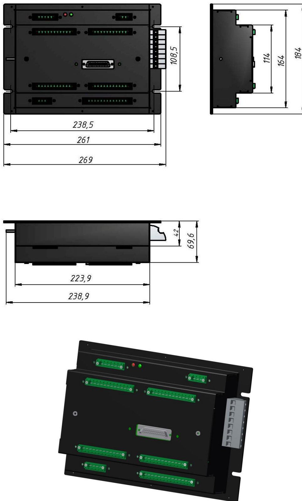
Рисунок К.1 – Внешний вид и габаритный чертеж блока защиты
