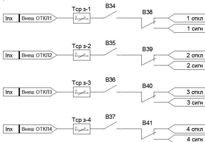
Рисунок 1.6.13 – Функциональная схема отключений от внешних защит
