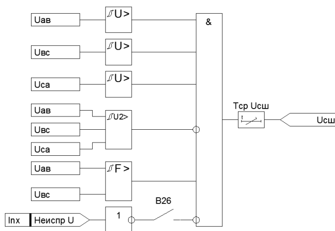
Рисунок 1.6.15 – Функциональная схема формирования U сш
