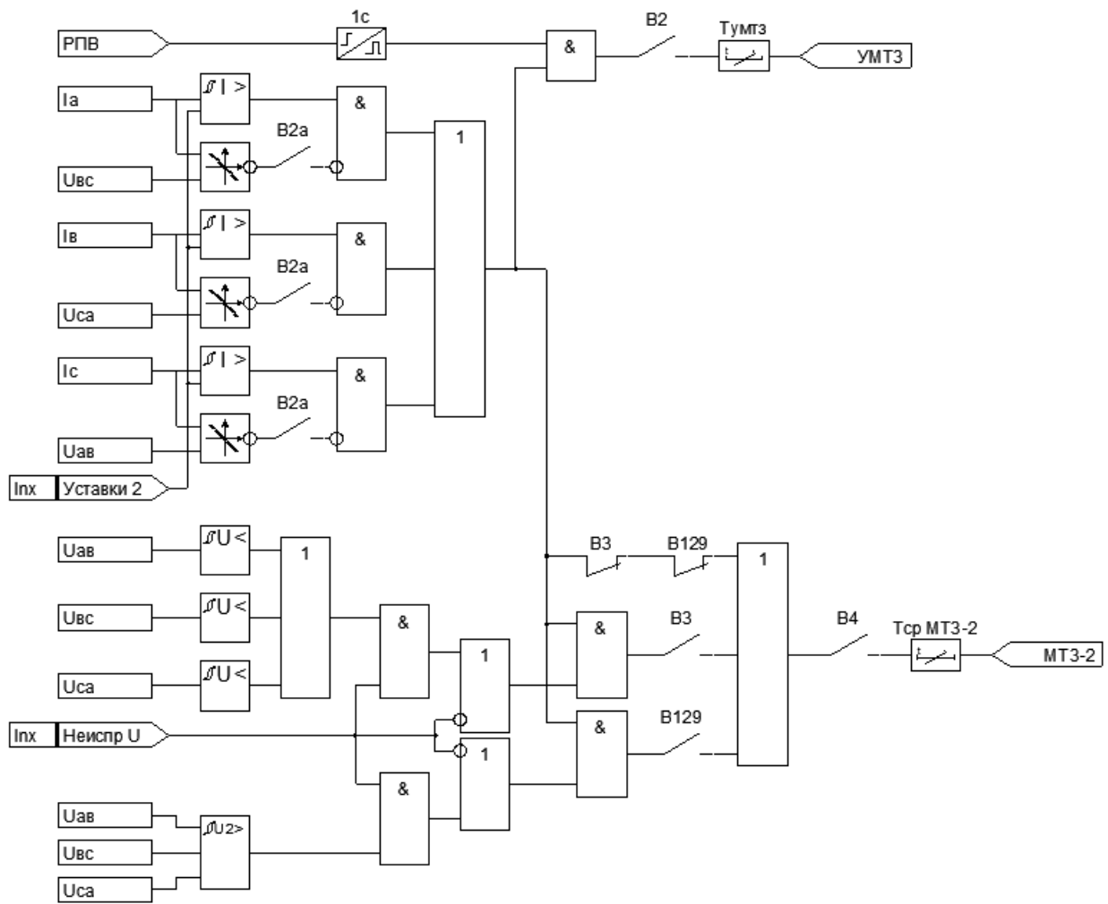
Рисунок 1.6.1.б – Функциональная схема МТЗ-2
