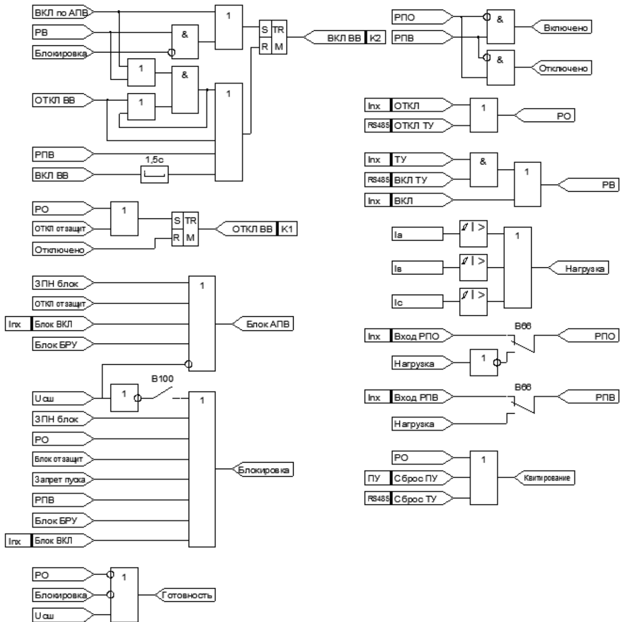
Рисунок 1.6.16 – Функциональная схема логики управления выключателем ОТ
