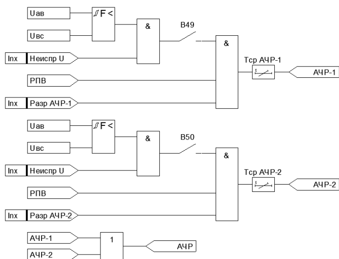
Рисунок 1.6.14 – Функциональная схема АЧР
