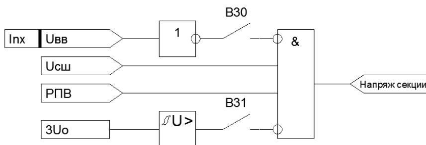
Рисунок 1.6.24 – Функциональная схема формирования сигнала «Увстр» для соседней секции шин
