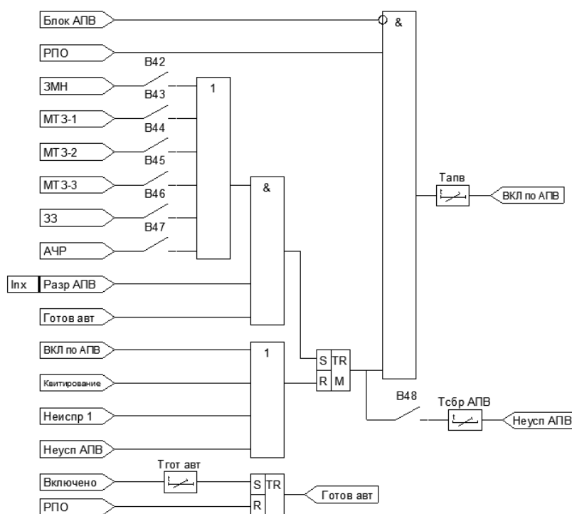
Рисунок 1.6.11 – Функциональная схема АПВ
