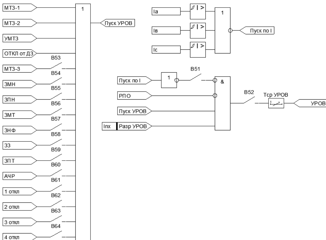
Рисунок 1.6.12 – Функциональная схема УРОВ
