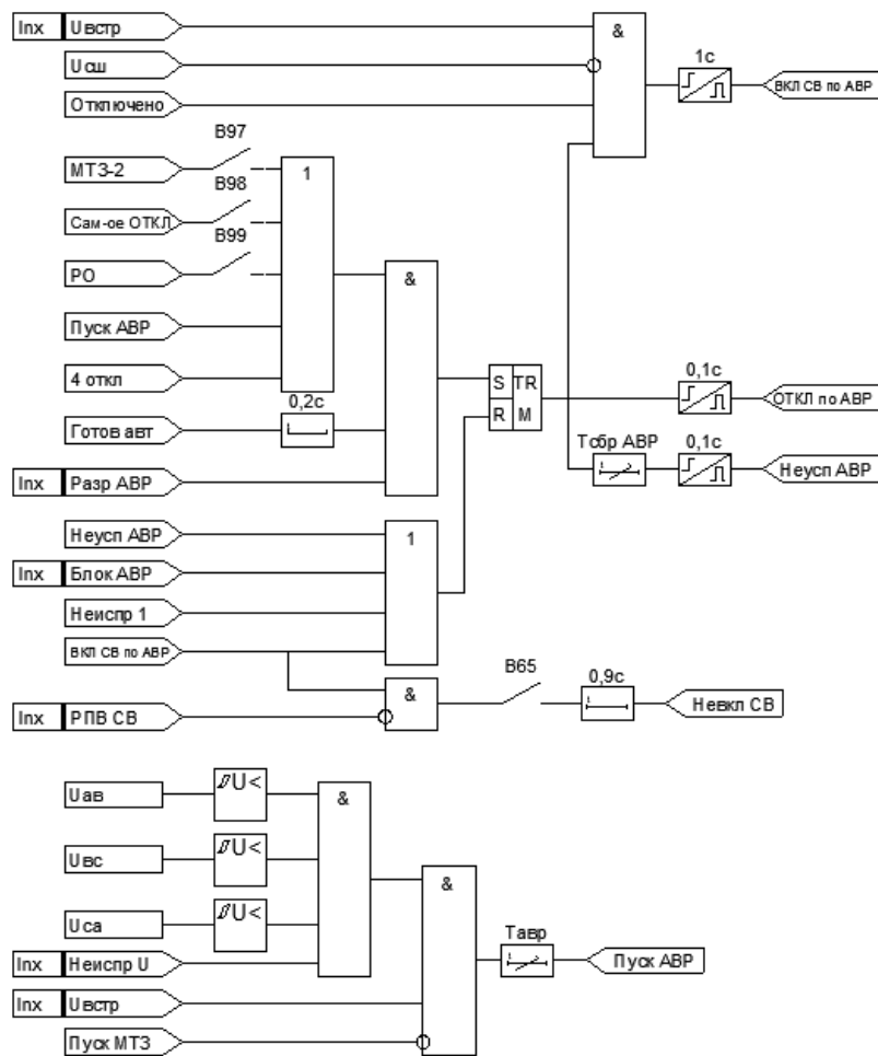
Рисунок 1.6.23 – Функциональная схема АВР ВВ
