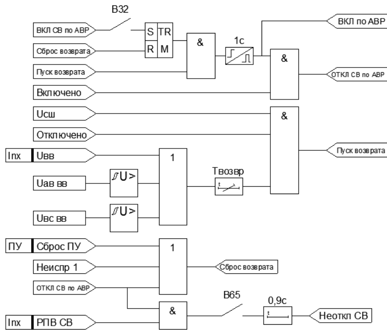
Рисунок 1.6.25 – Функциональная схема возврата после АВР
