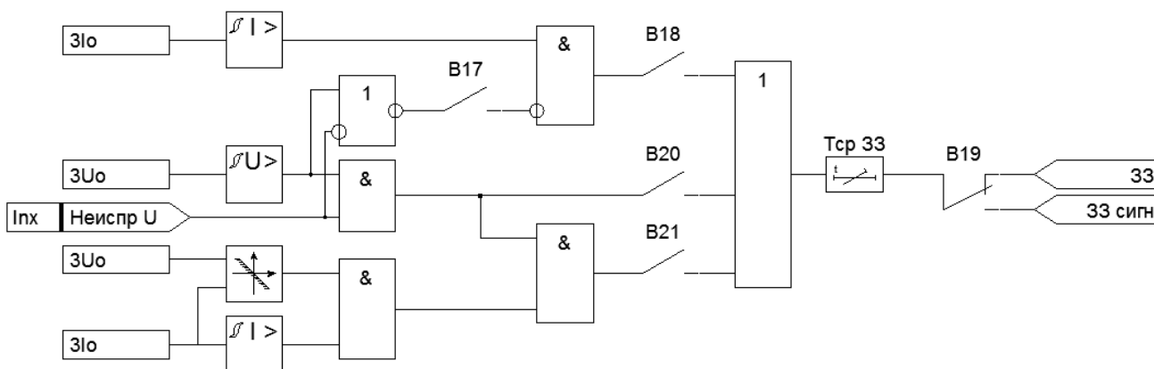
Рисунок 1.6.3 – Функциональная схема ЗЗ
