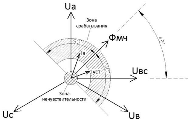
Рисунок 4.1.2 - Определение направления мощности
