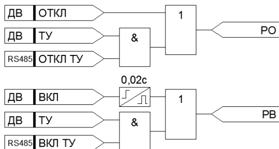
Рисунок 4.3.4 – Функциональная схема ручного управления ВВ при настройке «МУ» как «всегда 0»
