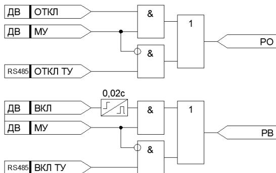
Рисунок 4.3.3 – Функциональная схема ручного управления ВВ при приоритете ДВ «МУ»
