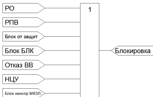
Рисунок 4.3.8 – Функциональная схема формирования сигнала блокировки РВ
