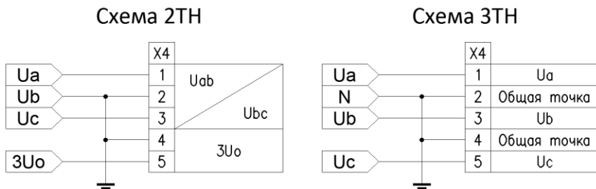
Рисунок 3.1 – Варианты подключения цепей напряжения
