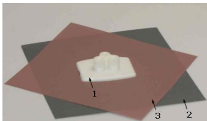
Рисунок 5.4 - Оправка (1), шлифовальная бумага с зернистостью "600" (2), полировальная пленка (3)
