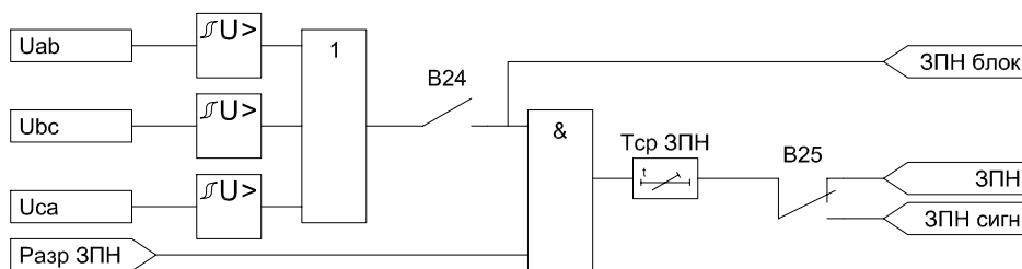
Рисунок 5.1.10 – Функциональная схема ЗПН
