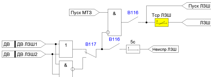
Рисунок 4.1.21 – Функциональная схема ЛЗШ
