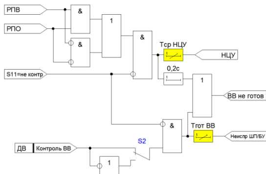
Рисунок 4.4.1 – Функциональная схема формирования сигналов «НЦУ», «неиспр ШП/БУ» и «ВВ не готов»
