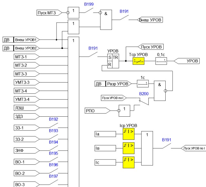
Рисунок 4.2.12 – Функциональная схема УРОВ
