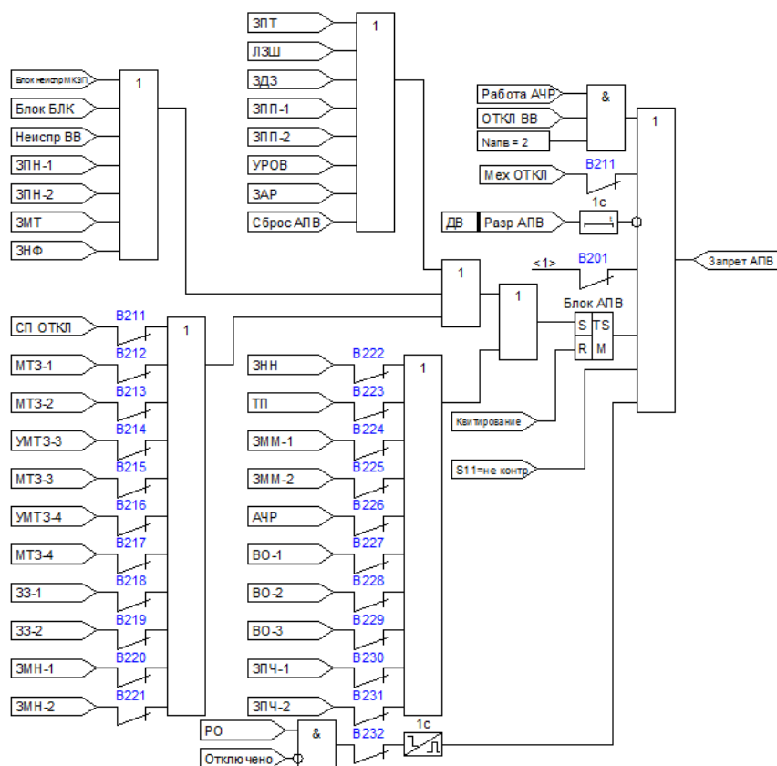
Рисунок 4.2.4 – Функциональная схема формирования сигнала запрета АПУ
