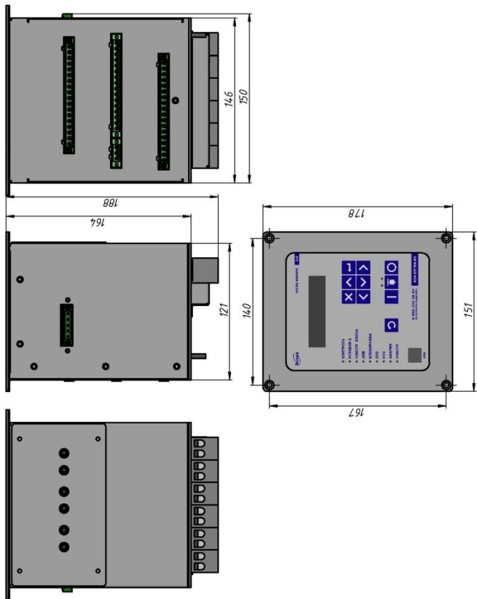
Габаритный чертеж корпуса в модификациях: 2.0-2-Т, 2.0-2-ДШ, 2.0-2-ДЗ, 2.0-2-Т-ДЗ, 2.0-2-ДШ-ДЗ, 2.0-3, 2.0-3-Т, 2.0-3-ДШ, 2.0-3-ДЗ, 2.0-4
