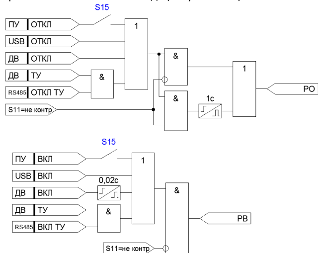
Рисунок 4.3.4 – Функциональная схема ручного управления ВВ при настройке «МУ» как «всегда 0»
