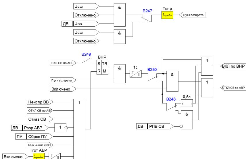
Рисунок 4.2.3 – Функциональная схема ВНР
