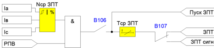
Рисунок 4.1.18 – Функциональная схема ЗПТ
