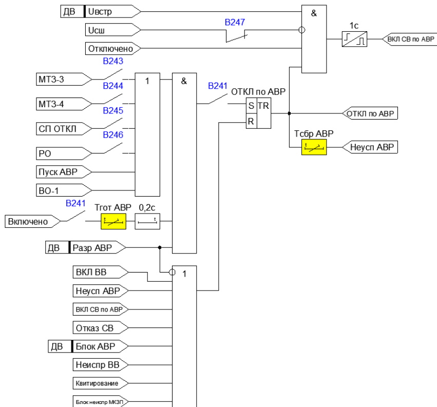
Рисунок 4.2.1 – Функциональная схема АВР
