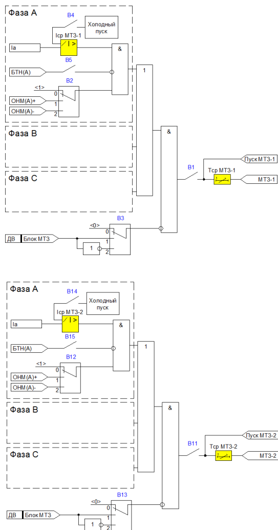
Рисунок 4.1.1 – Функциональная схема МТЗ-1 и МТЗ-2
