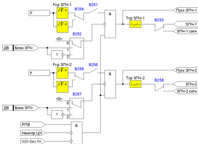
Рисунок 4.1.32 – Функциональная схема ЗПЧ для сервисной уставки «Тип присоединения» = ОЛ, ВВ
