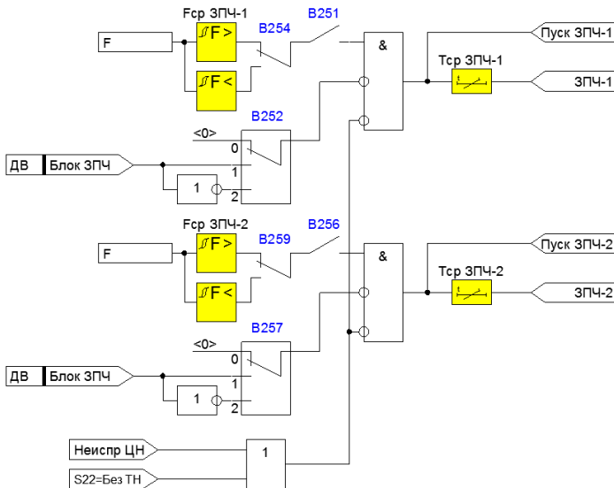
Рисунок 4.1.32 – Функциональная схема ЗПЧ для сервисной уставки «Тип присоединения» = ОЛ, ВВ
