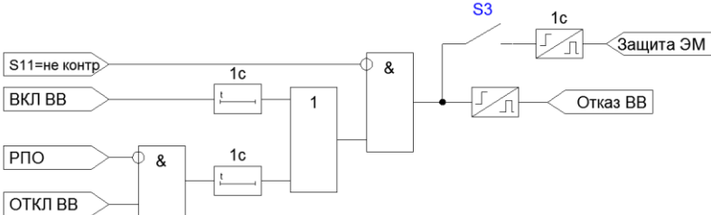
Рисунок 4.4.2 – Функциональная схема формирования сигнала отказа ВВ
