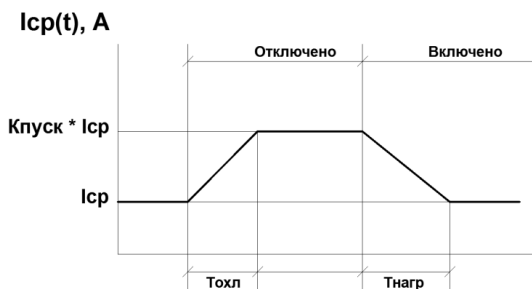
Рисунок 4.1.3 – Функция учета холодного пуска нагрузки
