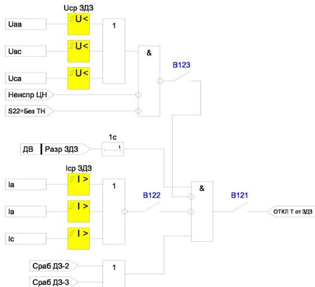
Рисунок 4.1.27 – Формирование сигнала «ОТКЛ Т от 3ДЗ» для сервисной уставки «Тип присоединения» = ВВ
