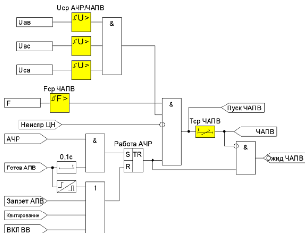
Рисунок 4.2.10 – Функциональная схема ЧАПВ
