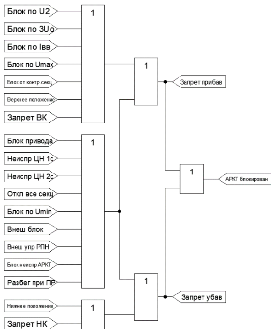
Рисунок 4.5.1 – Функциональная схема формирования сигналов запрета прибавить и убавить
