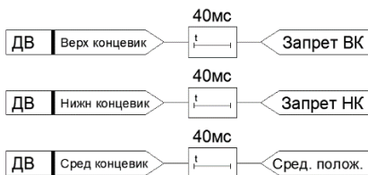
Рисунок 4.5.6 – Функциональная схема формирования сигналов блокировок от конечных выключателей приводного механизма
