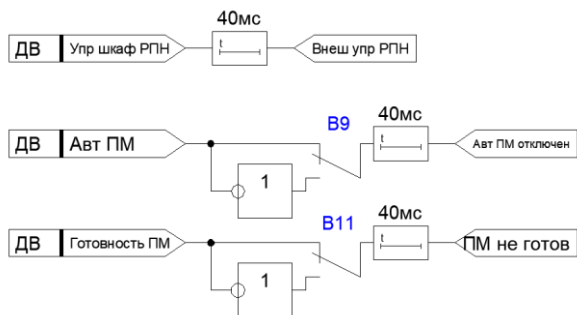
Рисунок 4.5.4 – Функциональная схема блокировок от шкафа привода РПН
