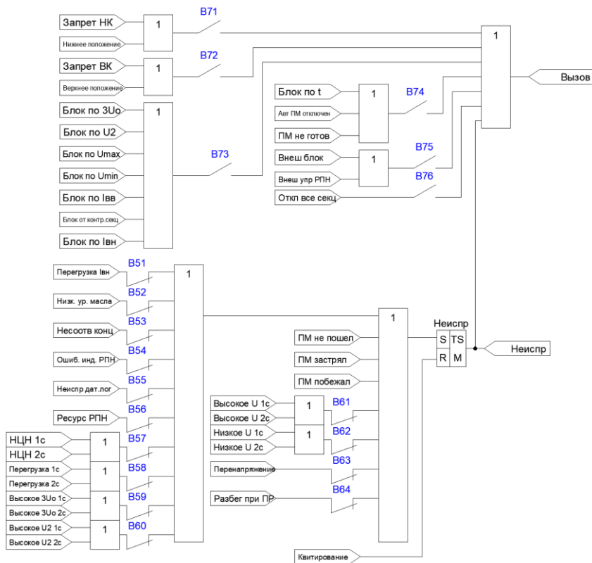
Рисунок 4.10.1 – Функциональная схема формирования сигналов сигнализации
