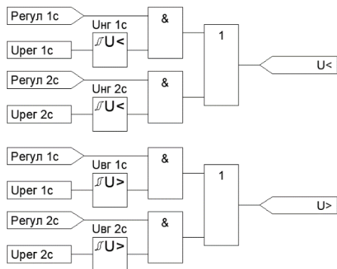
Рисунок 4.3.3 – Функциональная схема контроля выхода напряжения регулирования за зону нечувствительности
