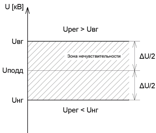
Рисунок 4.3.1 – Определение зоны нечувствительности при отсутствии встречного регулирования
