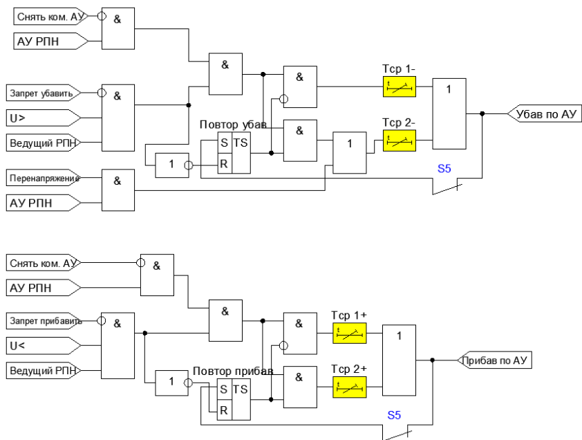
Рисунок 4.6.5 – Функциональные схемы формирования команд управления в автоматическом режиме при наличии параллельного регулирования
