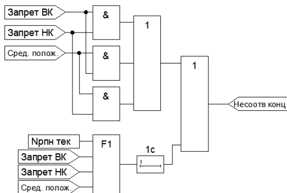
Рисунок 4.8.2 – Функциональная схема диагностики неисправности концевых выключателей
