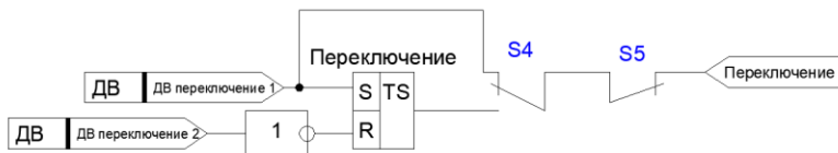
Рисунок 4.6.1 – Функциональные схемы формирования сигнала переключения
