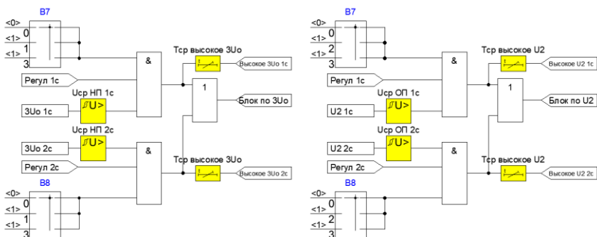
Рисунок 4.5.9 – Функциональные схемы формирования сигналов блокировки при несимметрии напряжений
