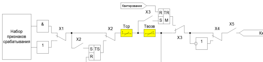
Рисунок 4.12.1 – Функциональная схема логики свободно программируемого реле
