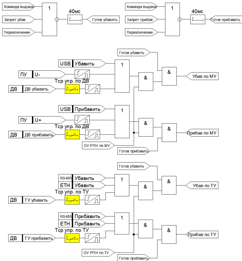
Рисунок 4.6.3 – Функциональные схемы формирования команд управления
