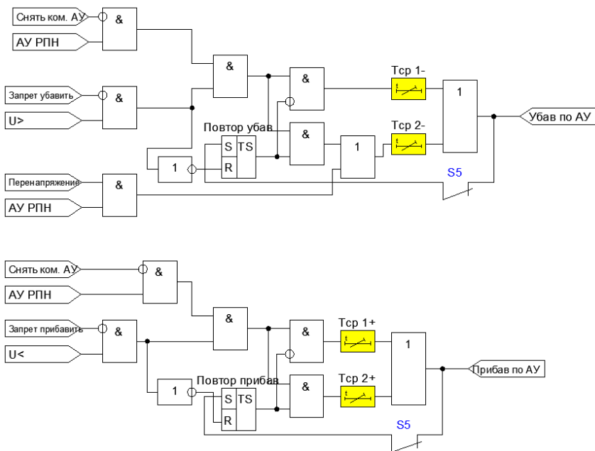
Рисунок 4.6.4 – Функциональные схемы формирования команд управления в автоматическом режиме при отсутствии параллельного регулирования
