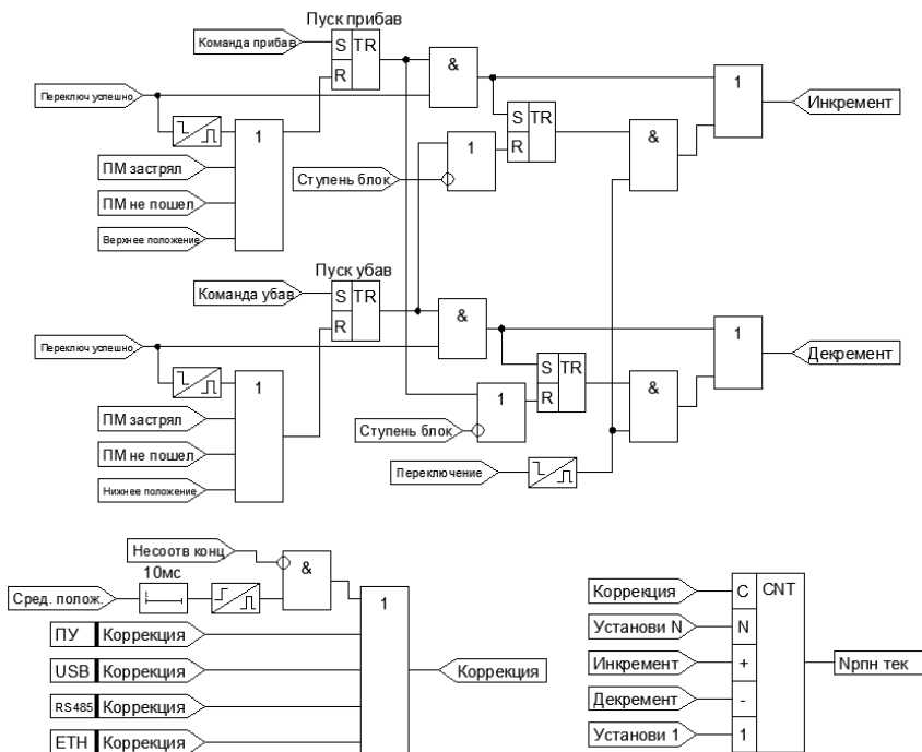
Рисунок 4.7.1 – Функциональная схема работы счетчика текущей ступени РПН
