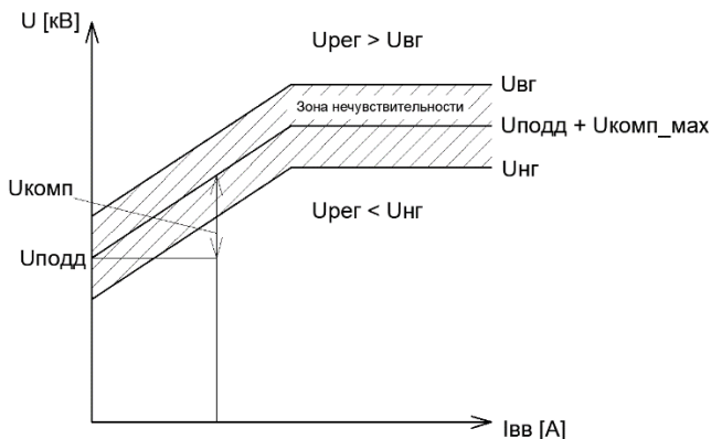
Рисунок 4.3.2 – Определение зоны нечувствительности при встречном регулировании
