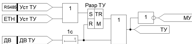
Рисунок 4.4.2 – Функциональная схема переключения режимов МУ и ТУ
