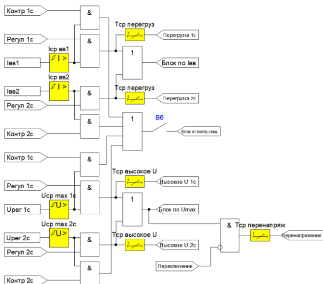
Рисунок 4.5.7 – Функциональная схема формирования блокировок от измеряемых сигналов тока и напряжения
