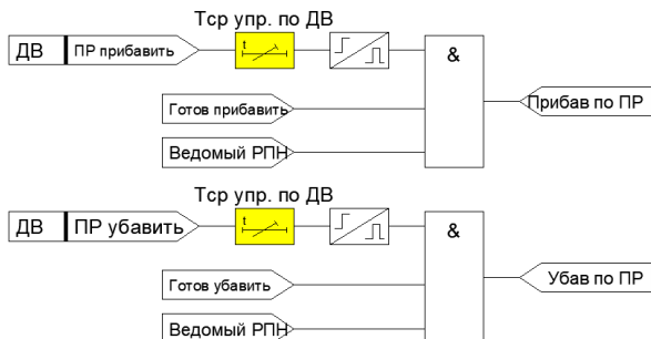
Рисунок 4.6.6 – Функциональная схема приема команд ведомым в режиме параллельного регулирования
