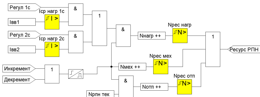
Рисунок 4.18.1 – Функциональная схема учета ресурса привода РПН
