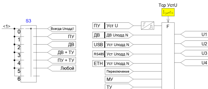
Рисунок 4.2.2 – Функциональная схема выбора текущего напряжения поддержания
