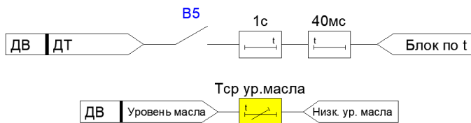
Рисунок 4.5.3 – Функциональная схема блокировки от датчика температуры и датчика низкого уровня масла
