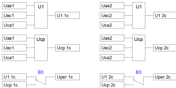
Рисунок 4.2.1 – Функциональная схема выбора типа регулируемого напряжения
