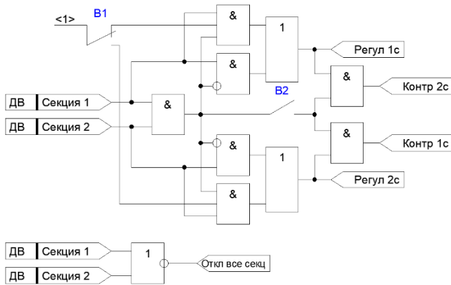
Рисунок 4.1.1 – Функциональная схема выбора регулируемой и контролируемой секций
