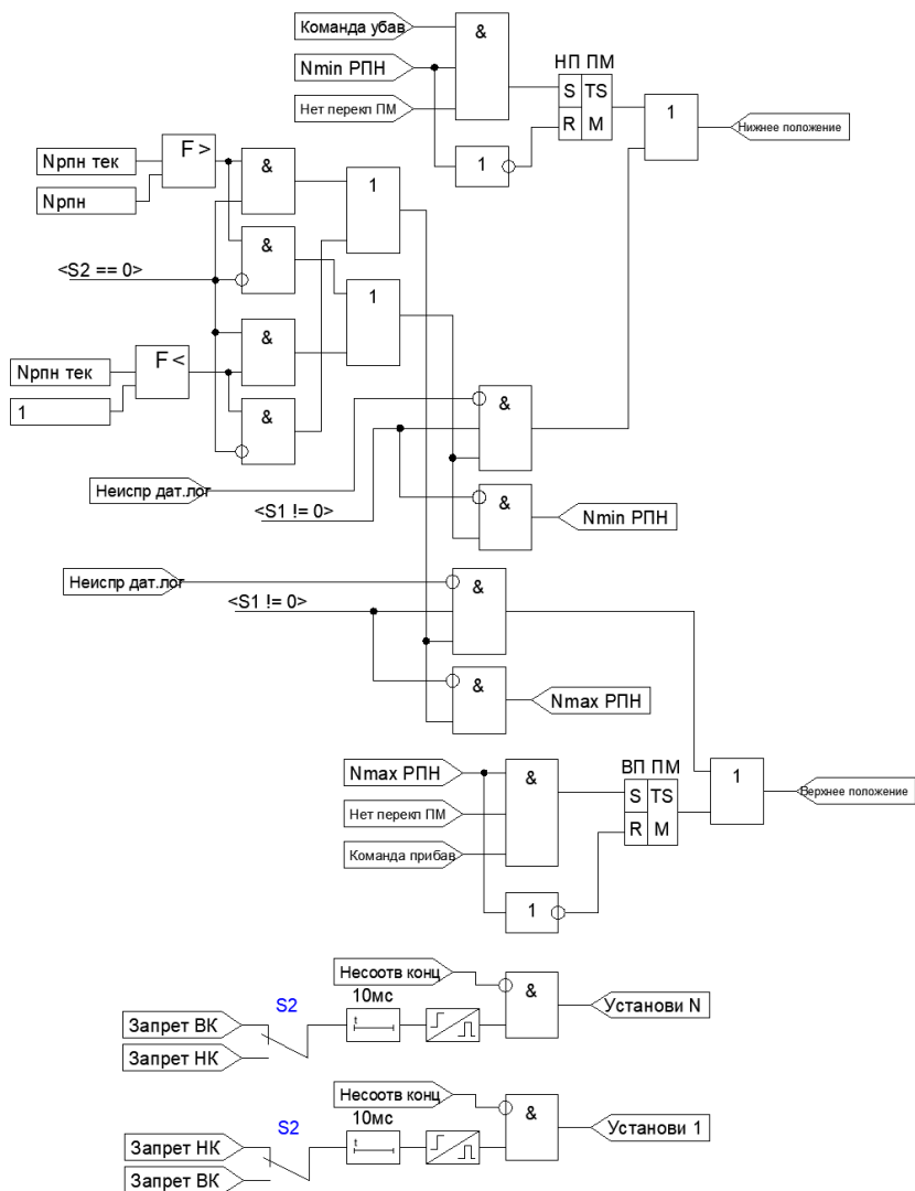
Рисунок 4.7.2 – Функциональная схема определения крайних ступеней РПН
