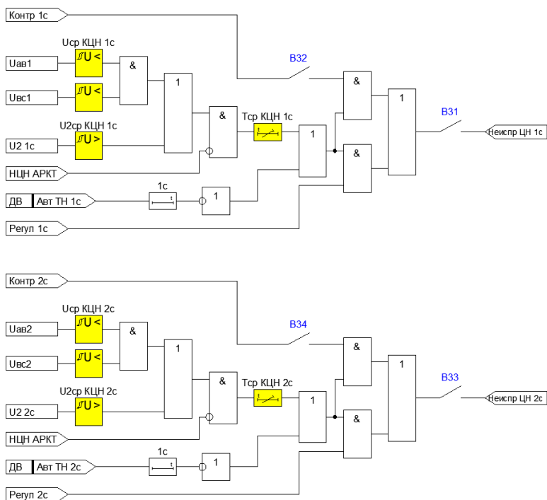
Рисунок 4.9.1 – Функциональная схема контроля исправности цепей напряжения
