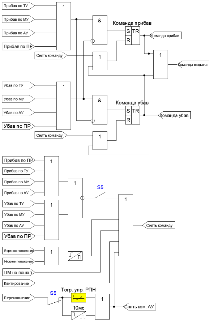
Рисунок 4.6.4 – Функциональные схемы формирования команд управления на привод РПН
