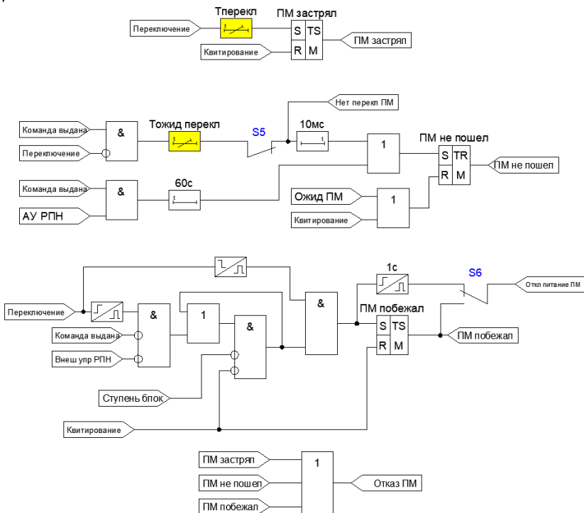
Рисунок 4.8.1 – Функциональная схема диагностики РПН
