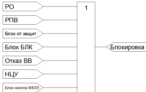
Рисунок 4.3.8 – Функциональная схема формирования сигнала блокировки РВ
