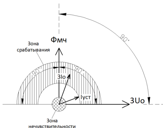
Рисунок 4.1.4 - Определение направления мощности нулевой последовательности
