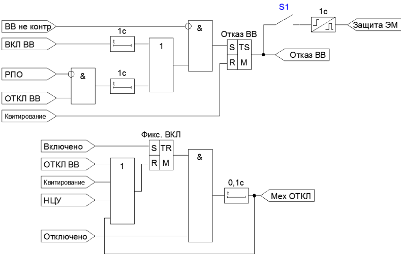
Рисунок 4.4.2 – Функциональная схема формирования сигнала отказа ВВ
